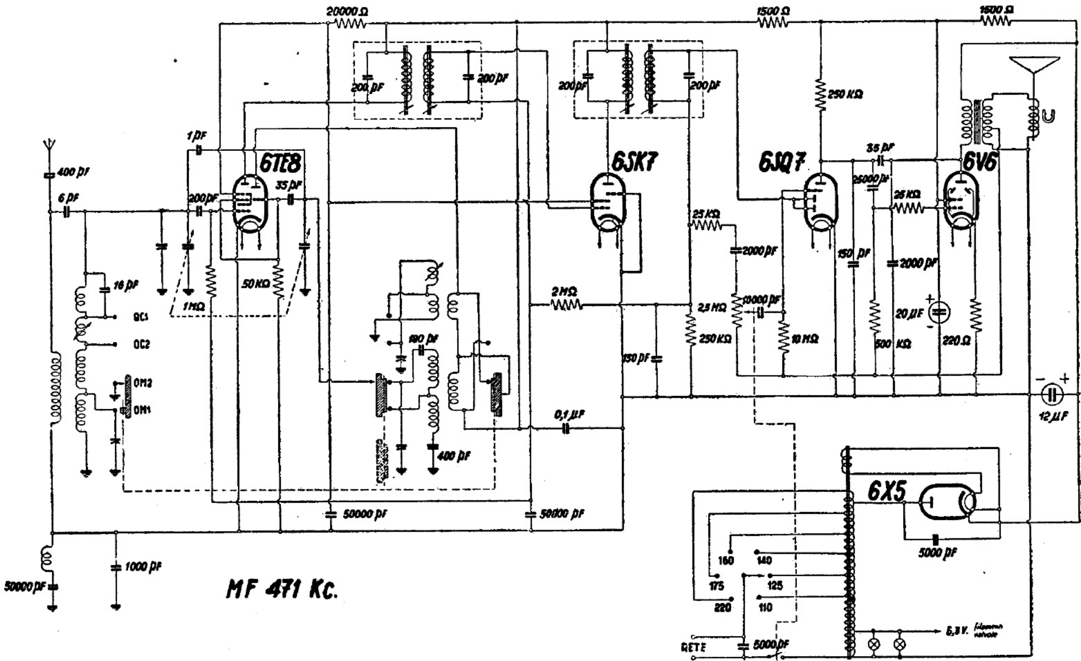
MAGNADYNE RADIO - Modd. S 22, S 23, S 24, S 32 e S 34 - Gamme medie e corte divise. Media frequenza 471 kc. Uscita 3 watt.
